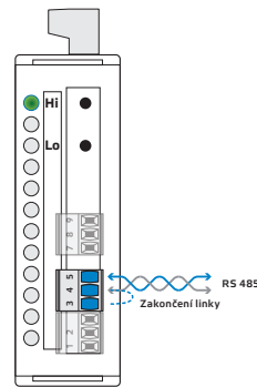
Datový výstup RS485
