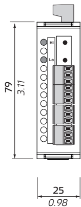
Pohled zepředu
