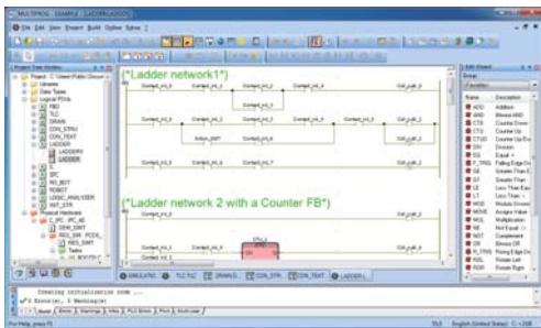
Рисунок 2: Диаграмма ступени
